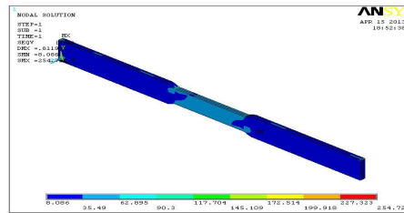
Von mises stress
