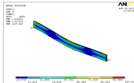
Von mises stress
